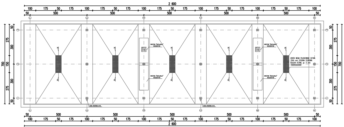
RZUT PŁYTY
