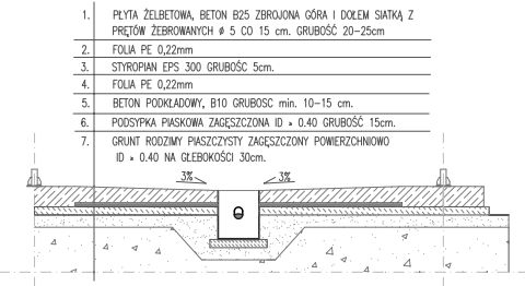
PRZEKRÓJ POSADZKI
