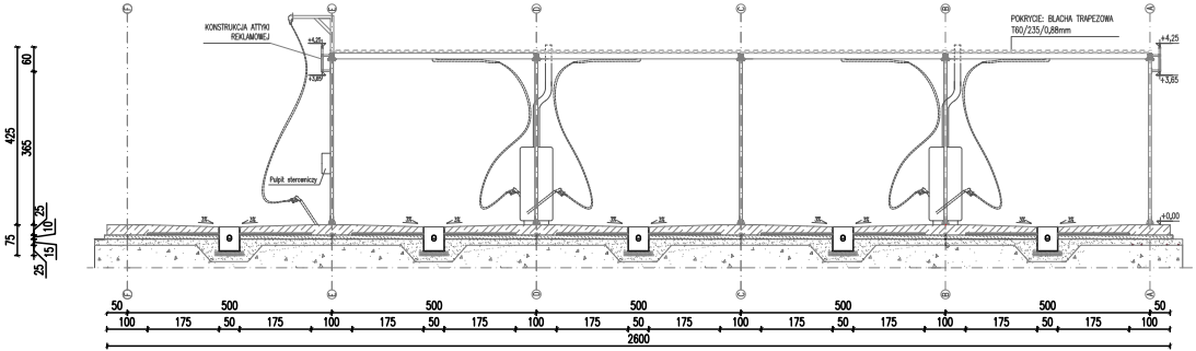
PRZEKRÓJ PODŁUŻNY
