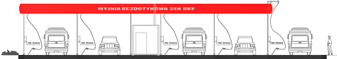
ELEWACJA FRONTOWA
