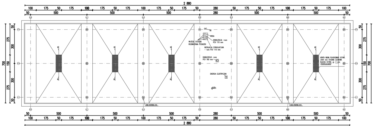
RZUT PŁYTY
