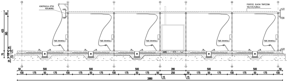
PRZEKRÓJ PODŁUŻNY
