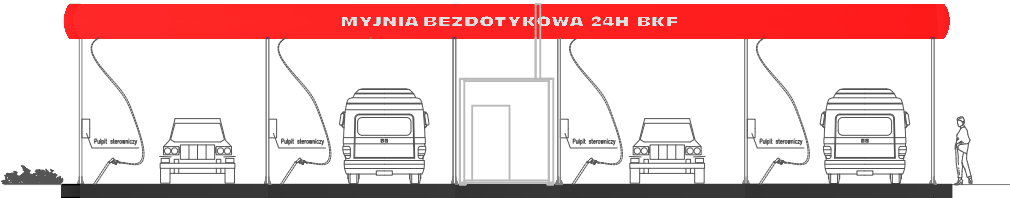
ELEWACJA FRONTOWA
