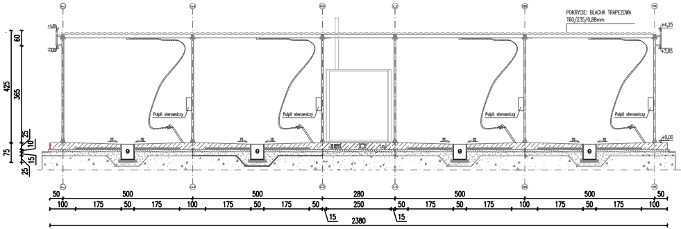
PRZEKRÓJ PODŁUŻNY
