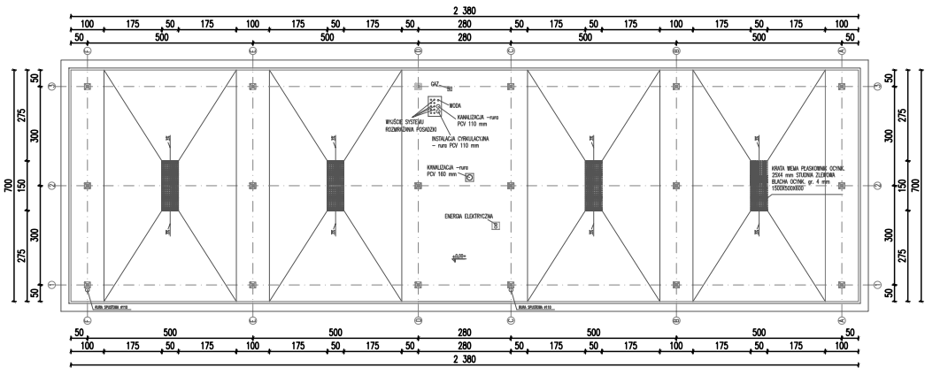
RZUT PŁYTY
