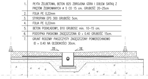
PRZEKRÓJ POSADZKI
